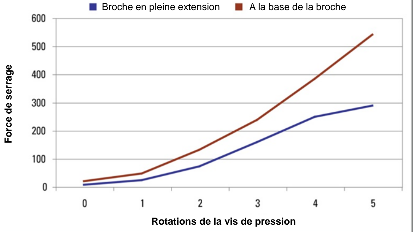
Génération de puissance de serrage du serre-joint à bascule de BESSEY
