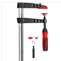
Skrutvting av aducerat gjutjärn med handtag av tvåkomponentmaterial TG-2K
