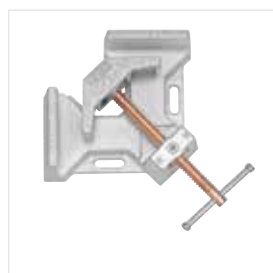
Hegesztők sarokszorítója
